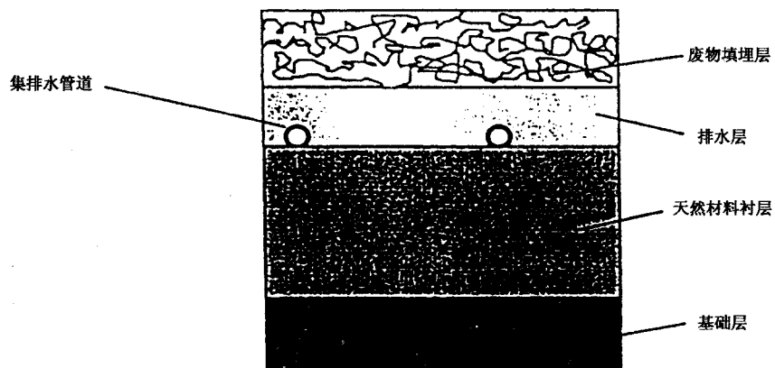
图 A.3 天然材料衬层示意图
